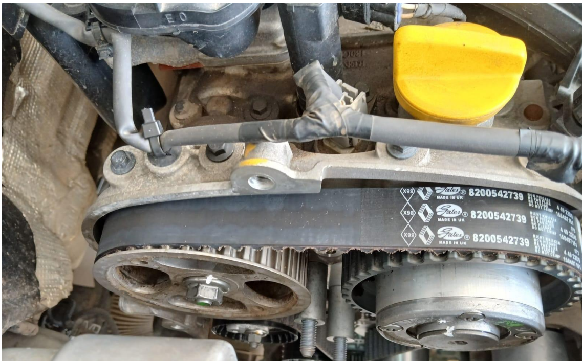
F6. Correa del kit de reparticion en su lugar
