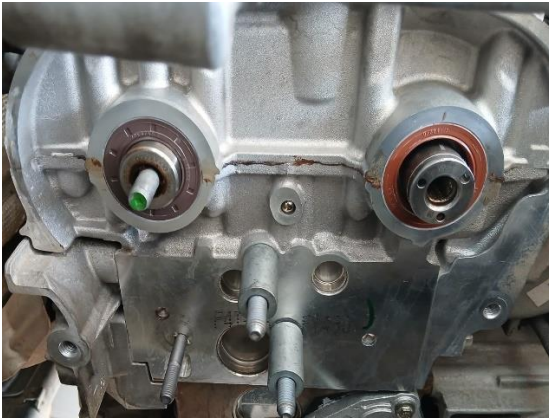
f4. Evidencia de los retendores nuevos instalados eje levas
